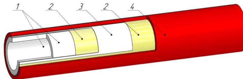
Рисунок 2 – Общий вид и конструкция изделия
